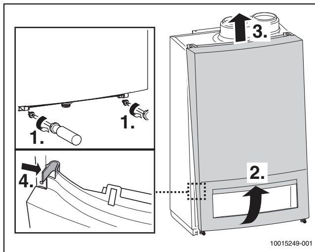
Afb. 26 Demonteren voorpaneel
