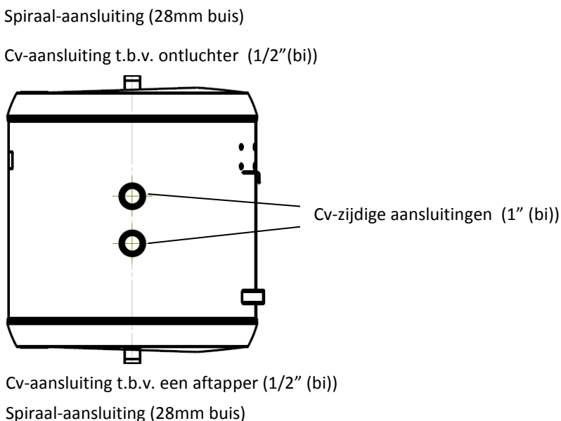
Achteraanzicht
