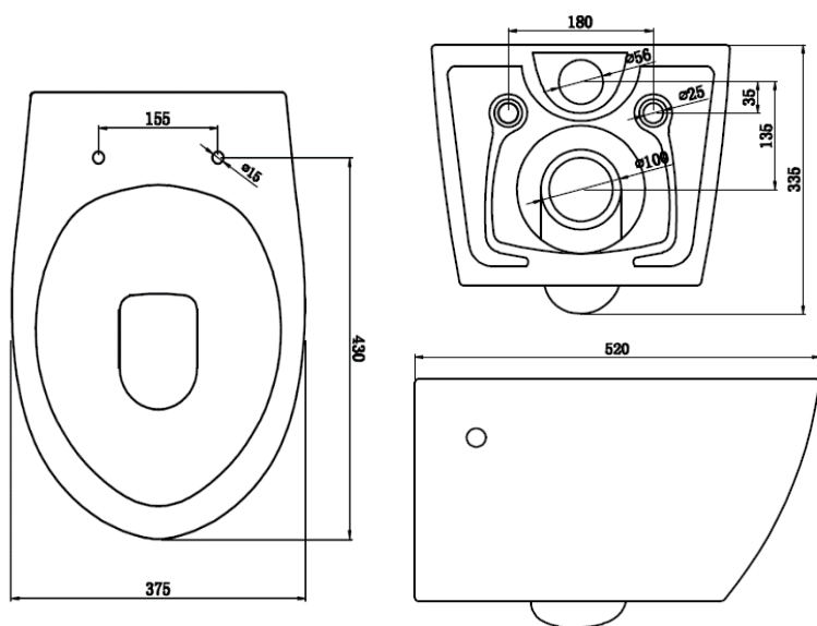
technische tekening / dessin technique
