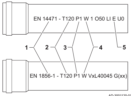
Afb.24 Voorbeelden tekenreeks
