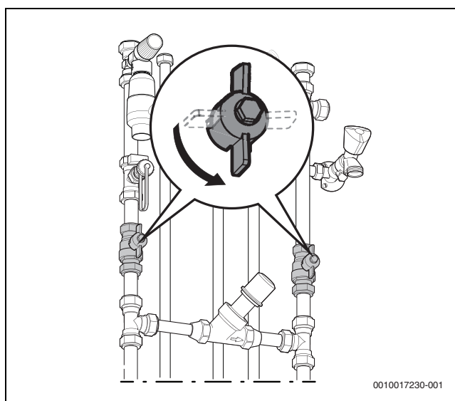
Afb. 4 Serviceafsluiters
