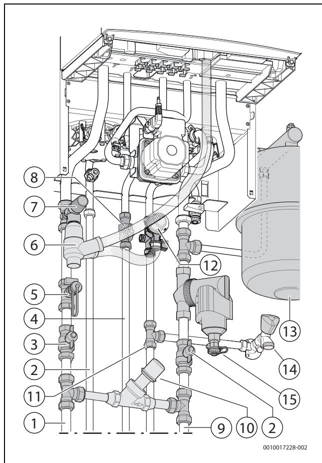
Afb. 2 Overzicht aansluitingen
