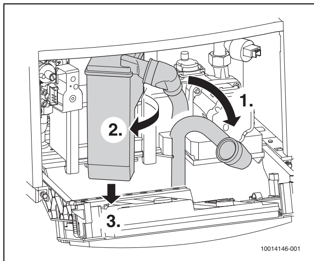
Afb. 48 Verwijderen toestelsifon
