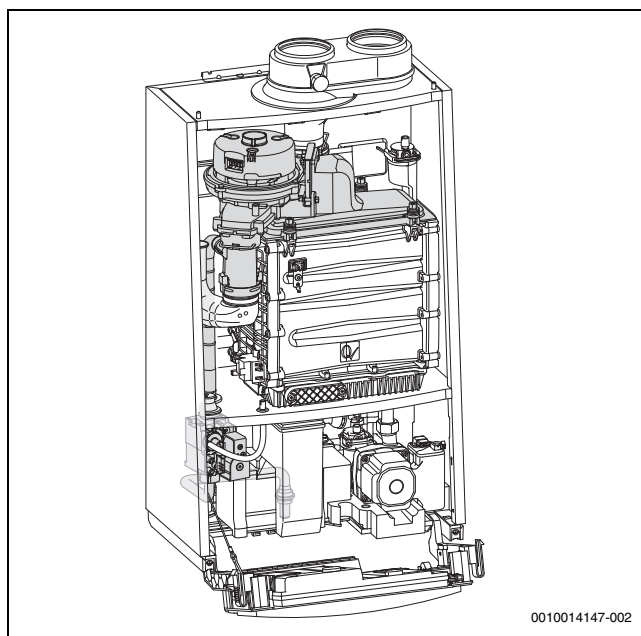
Afb. 54 Gasstraat
