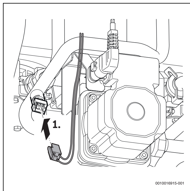
Afb. 35 Aansluiten inlaattemperatuursensor
