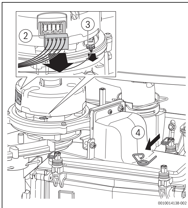
Afb. 43 Demonteren branderdekseel
