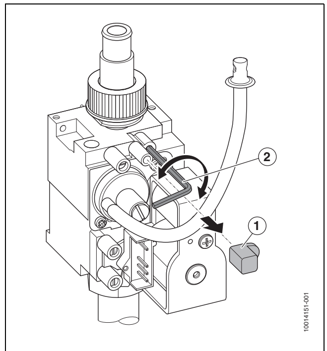
Afb. 59 Verstellen gasregelblok
