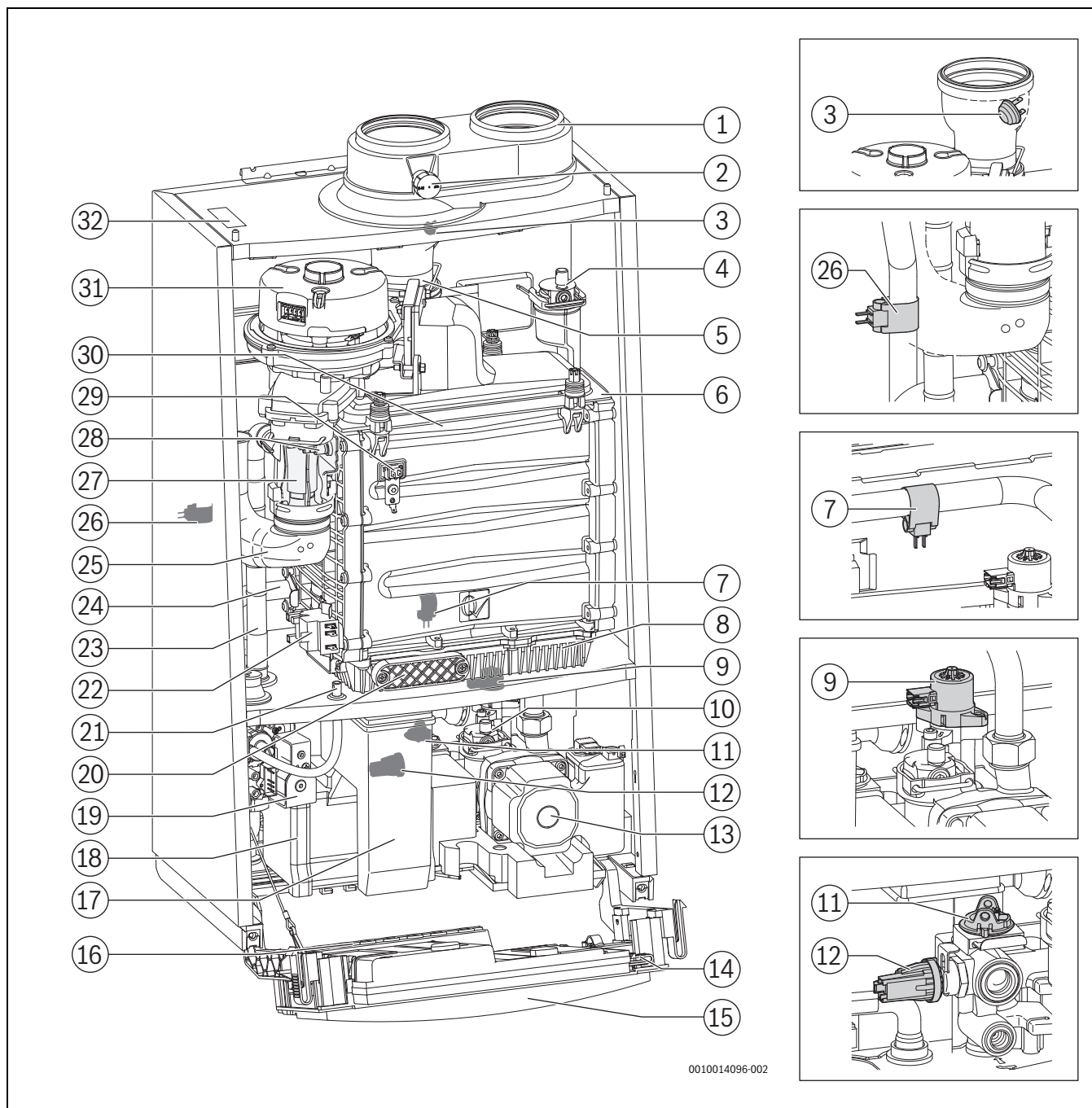
Afb. 1 Overzichtstekening
