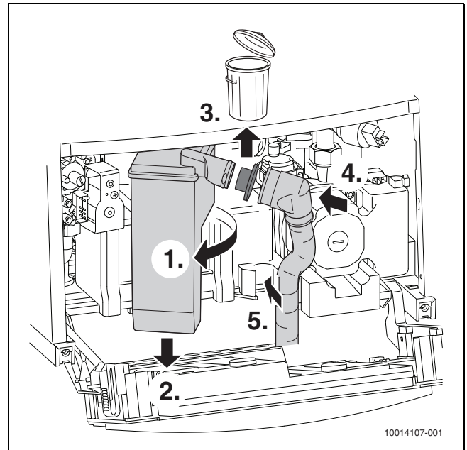
Afb. 19 Vullen toestelsifon
