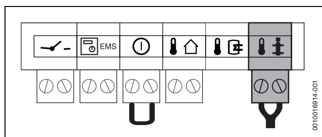
Afb. 34 Aansluiten inlaattemperatuursensor (bruin)
