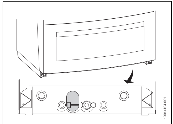
Afb. 14 Serviceopening warmwatertemperatuursensor
