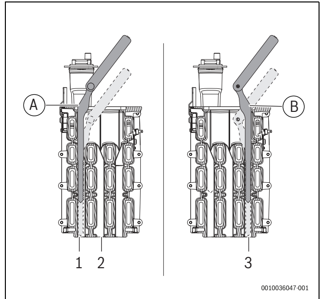
Afb. 46 Gebruik reinigingsmes
