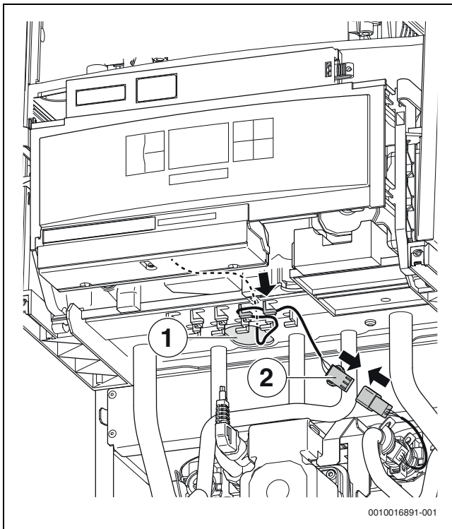
Afb. 18 Aansluiten flowsensor
