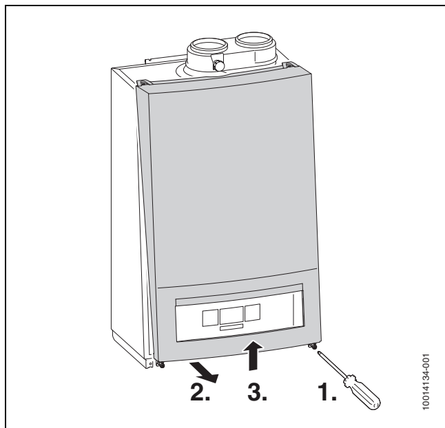
Afb. 41 Demonteren mantel
