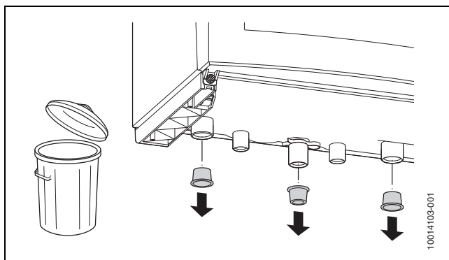
Afb. 13 Verwijderen beschermdoppen
