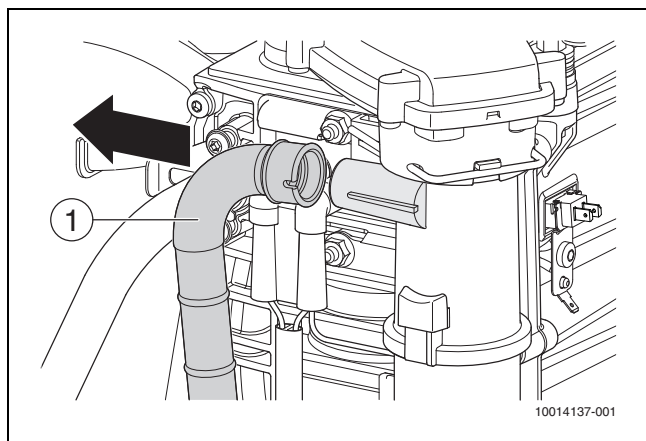
Afb. 42 Verwijderen gasslang
