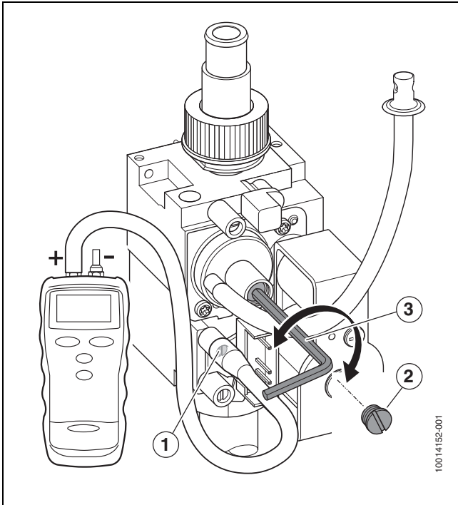
Afb. 60 Verwijderen afdekschroef en verdraaien stelschroef
