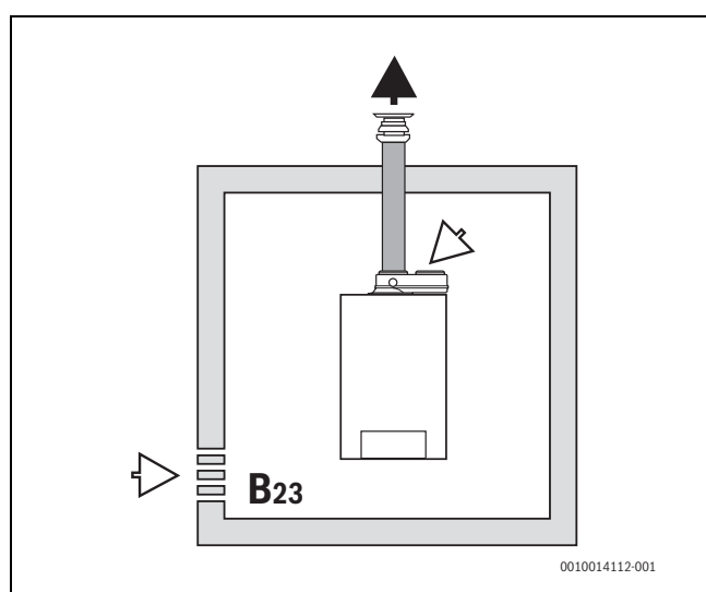
Afb. 5 Situatietekening rookgasafvoer type B 23
