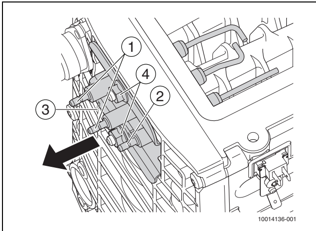
Afb. 45 Verwijderen ontstekingsunit
