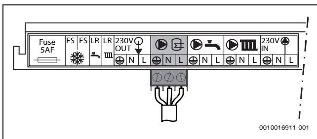
Afb. 27 Tapwaterpompaansluiting
