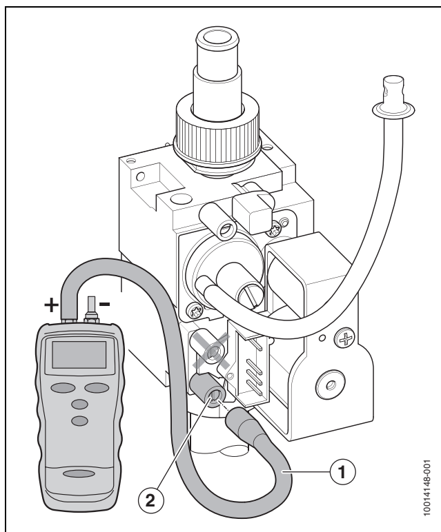
Afb. 56 Meten dynamische gasvoordruk
