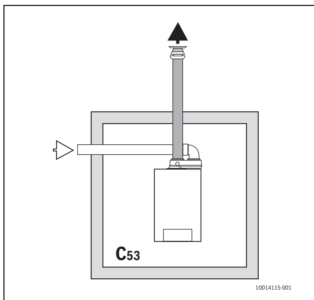
Afb. 9 Situatietekening rookgasafvoer type C 53
