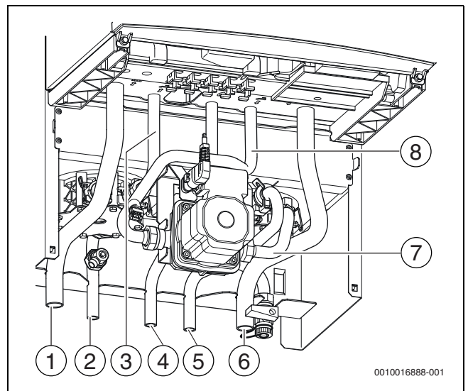
Afb. 15 Verbindingsstukken
