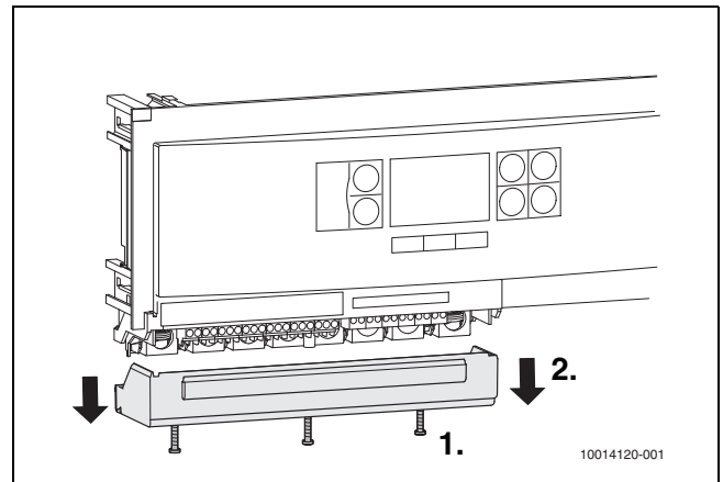
Afb. 24 Verwijderen beschermkap
