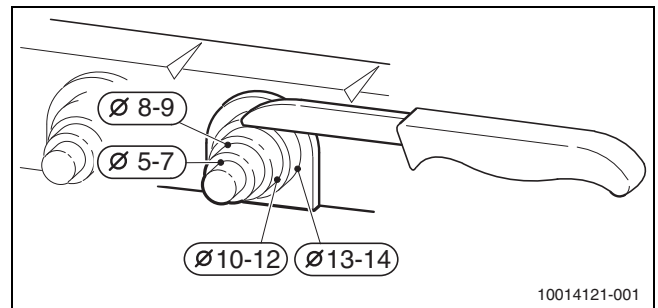
Afb. 25 Diameters kabeldoorvoeren
