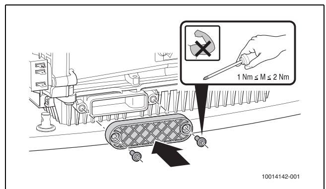
Afb. 47 Plaatsen servicedeksel
