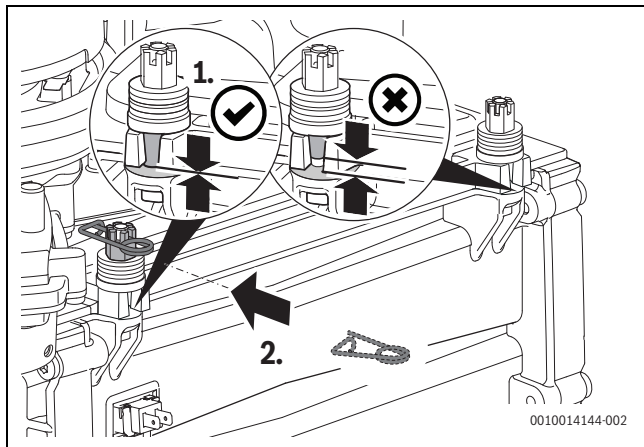
Afb. 52 Aandraaien moeren
