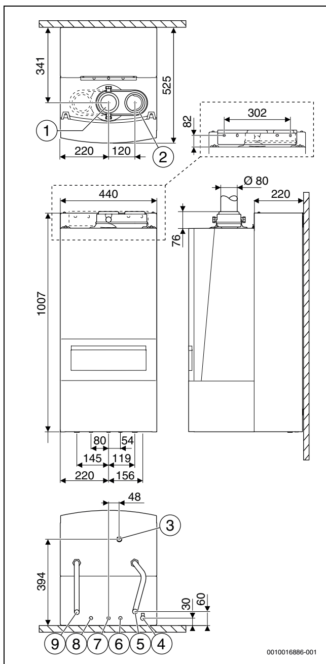
Afb. 4 Afmetingen [mm]
