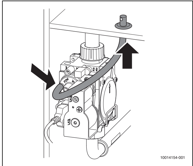
Afb. 62 Positie drukvereffeningsslang
