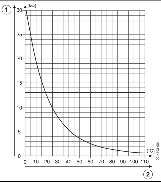
Afb. 66 Weerstandsgrafiek temperatuursensoren
