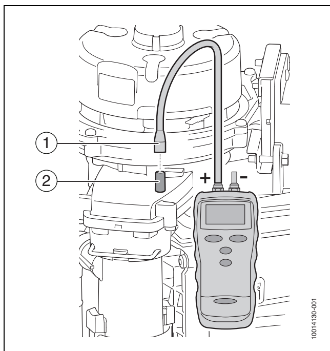
Afb. 55 Drukmeting
