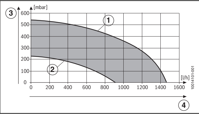
Afb. 65 Restopvoerhoogte cv-water
