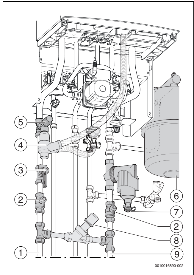
Afb. 17 Aansluiten cv-leidingen
