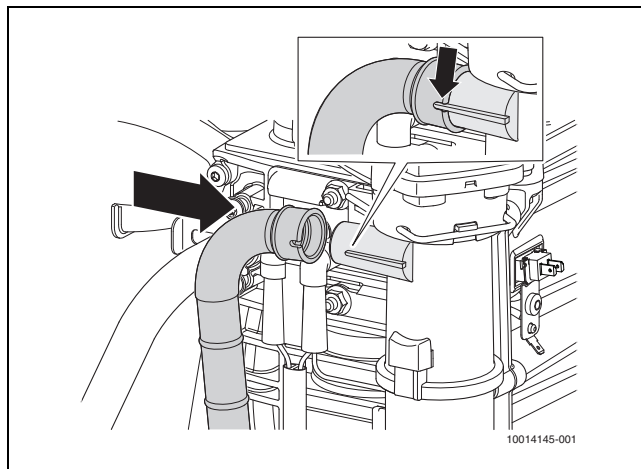
Afb. 53 Plaatsen gasslang
