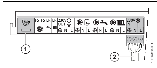
Afb. 28 Netspanningsaansluitingen
