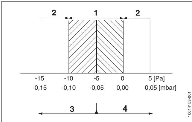
Afb. 61 Instellen drukverschil (op laaglast)
