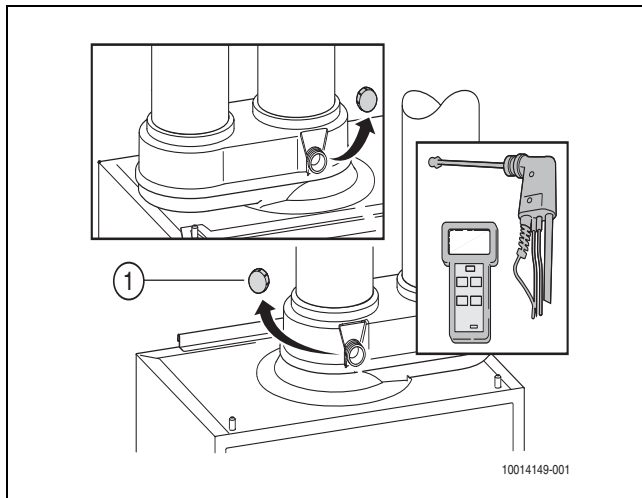
Afb. 57 Verwijderen afdekdop
