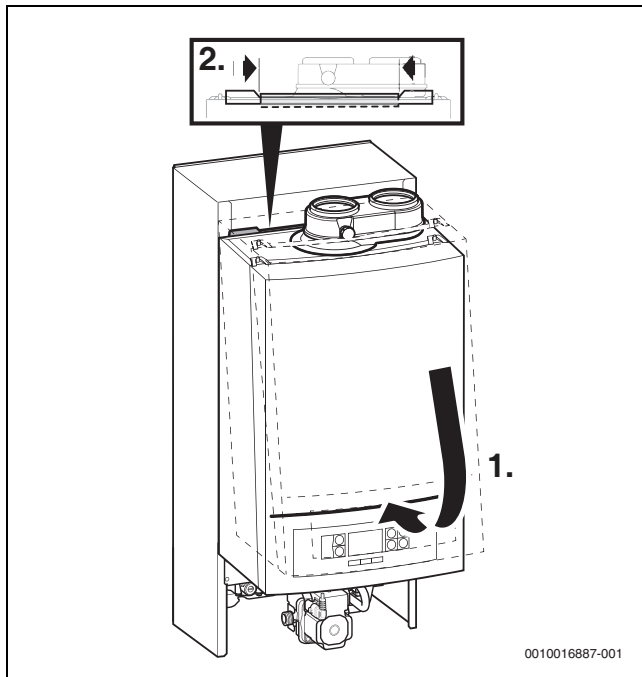
Afb. 12 Ophangen cv-toestel
