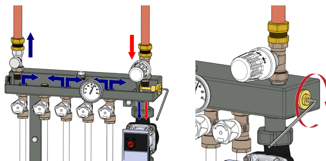
inregelventiel voor lage temperatuur toepassingen
